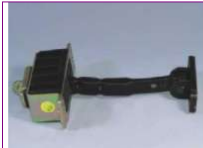
CW-DL-0015 BENZ W220 '98-03 DOOR CHECK ASSY 220 720 0016
